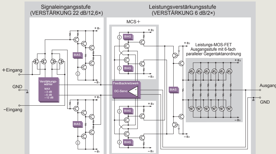
Schaltbild
